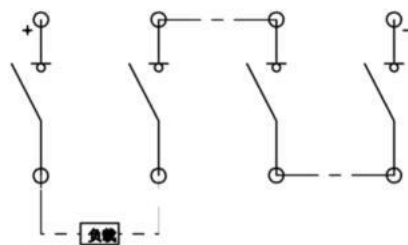
4P 外形接线图 (DC1000V)
