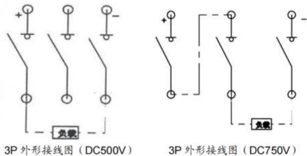
3P 外形接线图 (DC500V)
